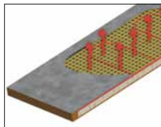
Section chauffage au sol
